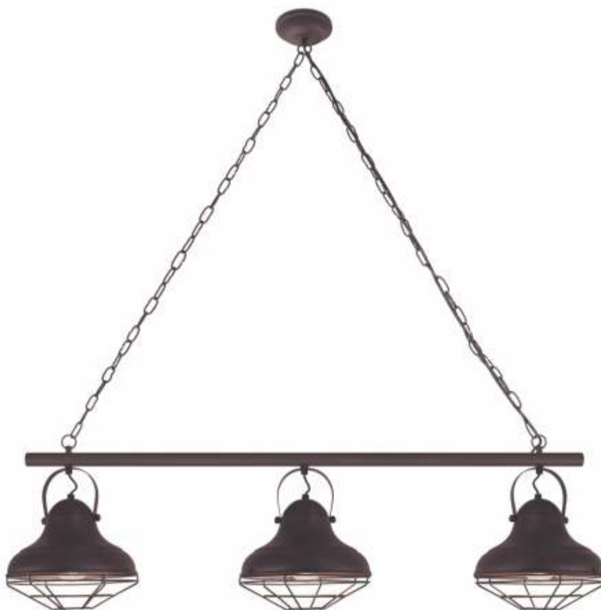
Pendente BARUC PLUS TRIPLO 1769 Porta lâmpada: 3 x E27 Luminária: Ø 1000 x 260 mm Base de teto: Ø 120 x 15 mm Cabo de alimentação: 1,5 m (regulável)
