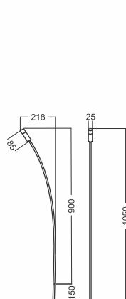
Balizador WAND 1435 Sem base Porta lâmpada: 1 x G9 Halopin Difusor: Acrílico fosco Luminária: Ø 25 x 85 mm Altura livre: 900 mm
