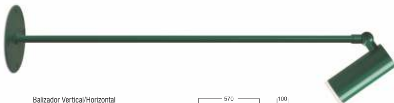
Balizador Vertical/Horizontal FIREFLY 1350 Com base Porta lâmpada: 1 x GU10 MR11 Difusor: Acrílico Spot: Ø 38 x 100 mm Base de piso/parede: Ø 100 x 2 mm Altura/Comprimento livre: 570 mm
