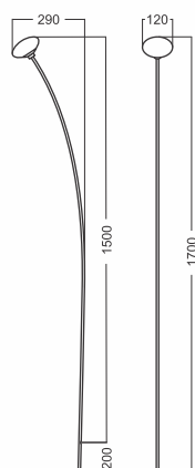
Balizador PAPOULA 1402 Sem base LED: 1 x 3W - 3000K 300 Lúmens - 127 V ou 220V Difusor: Globo amendoado de vidro branco opalino Ø 120 x 60 mm Luminária: Ø 120 x 70 mm Altura livre: 1500 mm
