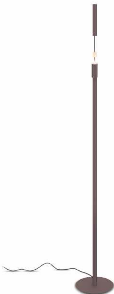
Coluna FLOAT 3015 Porta lâmpada: 1 x GU10 MR11 Difusor: Acrílico fosco Luminária: Ø 240 x 475 mm Base: Ø 240 x 10 mm Altura: 1800 mm Cabo de alimentação: 2,50 m (com interruptor de piso)
