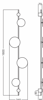
Arandela MOON 6097 Porta lâmpada: 4 x G9 Halopin Luminária: 70 x 340 x 1600 mm Base de parede: Ø 60 x 70 mm
