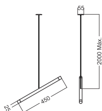
Pendente WAND PÊNDULO 2119 Porta lâmpada: 2 x G9 Halopin Difusor: Acrílico fosco Luminária: Ø 25 x 450 mm Base de teto: Full Contact Ø 55 x 3 mm Cabo de alimentação: 2 m (regulável)
