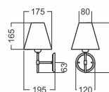
Arandela CHARLOTE METAL 1491 Porta lâmpada: 1 x E27 Cúpula em alumínio: Ø 175 x 165 mm Luminária: 195 x 175 x 310 Base de parede: Ø 120 x 15 mm
