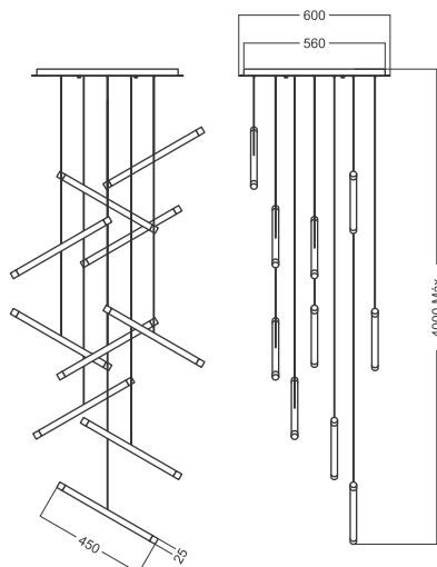
Pendente WAND PÊNDULO 2118 Porta lâmpada: 20 x G9 Halopin Difusor: Acrílico fosco Luminárias: Ø 25 x 450 mm Base de teto: Ø 560 x 25 mm c/ Blanket de Ø 600 mm Cabos de alimentação: 4 m (regulável)
