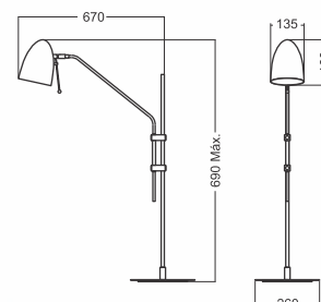
Abajur PISA 3525 Porta lâmpada: 1 x E27 Tamanho da cúpula: Ø 135 x 160 mm Altura máxima: 690 mm Alcance do braço: 670 mm Base: Ø 260 x 10 mm Cabo de alimentação: 1,80 m (com interruptor)
