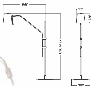
Abajur RAVENA POCO 3523 Porta lâmpada: 1 x E27 Tamanho da cúpula: Ø 125 x 125 mm Altura máxima: 690 mm Alcance do braço: 560 mm Base: Ø 260 x 8 mm Cabo de alimentação: 1,80 m (com interruptor)
