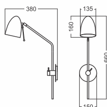
Arandela PISA 1484 Porta lâmpada: 1 x E27 Tamanho da cúpula: Ø 135 x 160 mm Altura máxima: 660 mm ( ajuste vertical e lateral ) Alcance do braço: 380 mm Base de parede: Ø 120 x 15 mm (Blanket Ø 150) Cabo de alimentação: 1,80 m (com interruptor)
