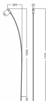
Balizador WAND 1437 Sem base Porta lâmpada: 1 x G9 Halopin Difusor: Acrílico fosco Luminária: Ø 25 x 85 mm Altura livre: 1500 mm
