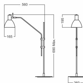
Abajur ROMA 3514 Porta lâmpada: 1 x E27 Tamanho da cúpula: Ø 165 x 195 mm Altura máxima: 690 mm Alcance do braço: 560 mm Base: Ø 260 x 8 mm Cabo de alimentação: 1,80 m (com interruptor)
