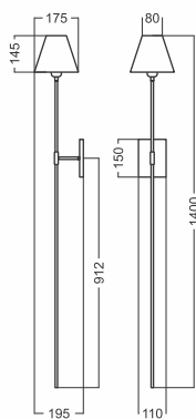
Arandela DINA 4040 Porta lâmpada: 1 x E27 Cúpula em tecido: Ø 175 x 145 mm Luminária: 195 x 175 x 1400 Base de parede: 110 x 15 x 150 mm
