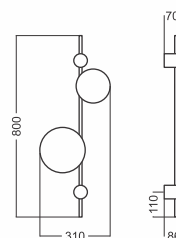
Arandela MOON 6117 Porta lâmpada: 2 x G9 Halopin Luminária: 70 x 310 x 800 mm Base de parede: Ø 60 x 70 mm
