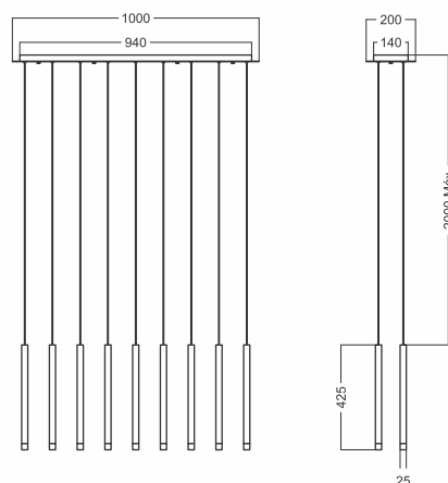
Pendente WAND BRT 2116 Porta lâmpada: 18 x G9 Halopin Difusor: Acrílico fosco Luminárias: Ø 25 x 425 mm Base de teto: 940 x 140 x 25 mm c/ Blanket de 1000 x 200 mm Cabos de alimentação: 2 m (regulável)
