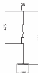
Abajur FLOAT 3527 Porta lâmpada: 1 x GU10 MR11 Difusor: Acrílico fosco Luminária: Ø 180 x 475 mm Base: Ø 180 x 10 mm Altura: 780 mm Cabo de alimentação: 1,80 m (com interruptor)
