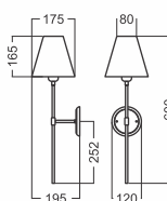
Arandela LUANA METAL 1620 Porta lâmpada: 1 x E27 Cúpula em alumínio: Ø 175 x 165 mm Luminária: 195 x 175 x 600 Base de parede: Ø 120 x 15 mm
