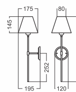
Arandela LUANA 4038 Porta lâmpada: 1 x E27 Cúpula em tecido: Ø 175 x 145 mm Luminária: 195 x 175 x 580 Base de parede: Ø 120 x 15 mm
