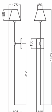
Arandela DINA METAL 1622 Porta lâmpada: 1 x E27 Cúpula em alumínio: Ø 175 x 165 mm Luminária: 195 x 175 x 1420 Base de parede: 110 x 15 x 150 mm
