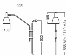
Arandela ROMA 4007 POCO BRACCIO Porta lâmpada: 1 x E27 Tamanho da cúpula: Ø 105 x 165 mm Altura ajustável: 555 mm Mín. / 710 mm Máx. Alcance do braço: 520 mm Bases de parede: Ø 25 x 25 mm Haste de parede: 555 mm Cabo de alimentação: 1,80 m (com interruptor)
