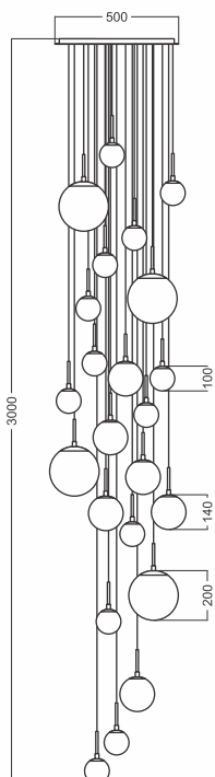
Pendente WASSERFALL 3M 1946 Porta lâmpada: 19 x G9 Halopin + 4 x E27 Difusores: Globos de vidro opalino branco 13 x Ø 100 mm 6 x Ø 140 mm 4 x Ø 200 mm Luminária: Ø 500 x 3000 mm Base de teto: Ø 500 x 20 mm Cabos de alimentação: 3 m (reguláveis)
