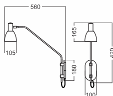
Arandela ROMA POCO BASE 1482 Porta lâmpada: 1 x E27 Tamanho da cúpula: Ø 105 x 165 mm Altura: 420 mm Alcance do braço: 560 mm Base de parede: 100 x 180 x 15 mm
