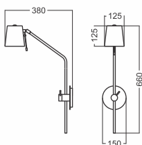
Arandela RAVENA POCO 4011 Porta lâmpada: 1 x E27 Tamanho da cúpula: Ø 125 x 125 mm Altura máxima: 660 mm (ajuste vertical e lateral) Alcance do braço: 380 mm Base de parede: Ø 120 x 15 mm c/ blanket de Ø 150 mm Cabo de alimentação: 1,80 m (com interruptor)
