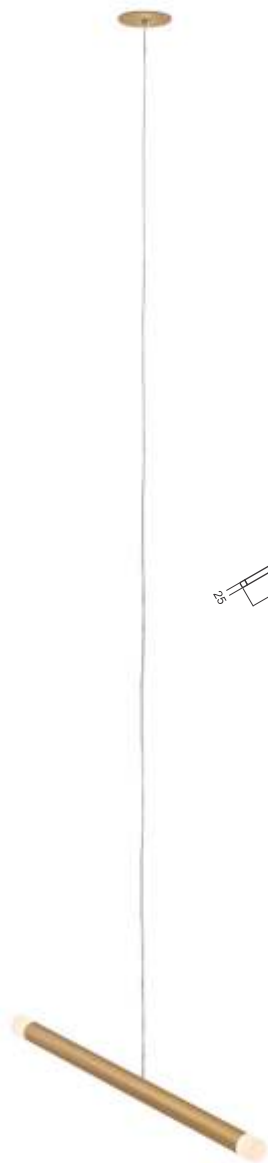
Pendente WAND PÊNDULO 2119 Porta lâmpada: 2 x G9 Halopin Difusor: Acrílico fosco Luminária: Ø 25 x 450 mm Base de teto: Full Contact Ø 55 x 3 mm Cabo de alimentação: 2 m (regulável)
