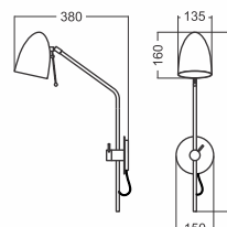
Arandela PISA UNO 1485 Porta lâmpada: 1 x E27 Tamanho da cúpula: Ø 135 x 160 mm Altura máxima: 660 mm ( ajuste vertical e lateral ) Alcance do braço: 380 mm Base de parede: Ø 120 x 15 mm (Blanket Ø 150)
